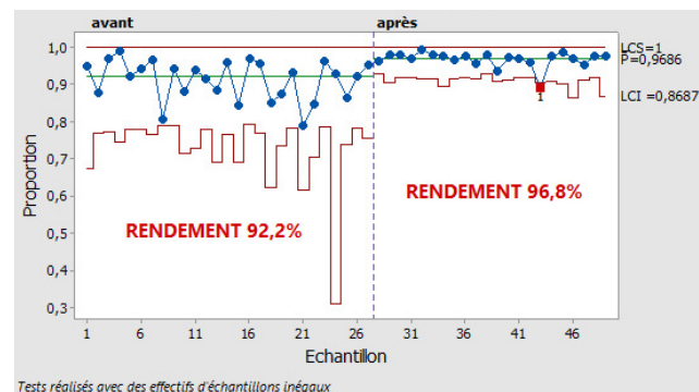
Carte P de Laney pour Q bonne totale (rendement global) Sigma Z = 8,5485;4,04749 Comparaison entre période d'observation de référence et après modification
