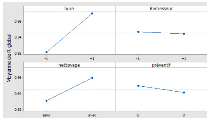
Graphique des effets principaux pour Rendement Global (moyennes ajustées)
